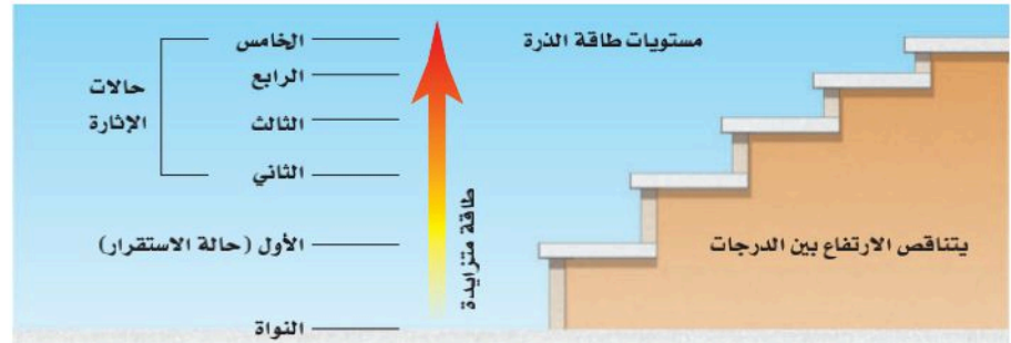
■ الشكل 10-4 هذه الدرجات التي يتناقص البعد بينها تماثل مستويات الطاقة المتاحة في الذرة. لاحظ كيف أن فرق الطاقة بين مستويات الطاقة المتجاورة يتناقص كلما زاد بعد مستوى الطاقة.
