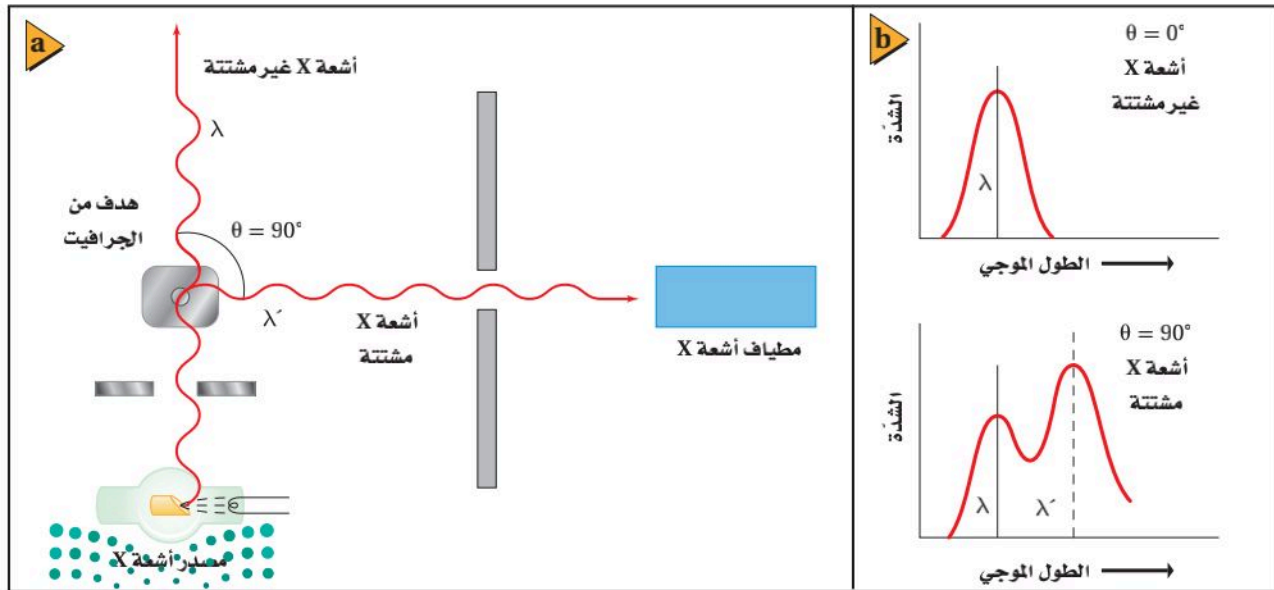
■ الشكل 3-6 استخدم كومبتون أدوات مشابهة لهذه الأدوات في دراسة طبيعة الفوتونات (a). زيادة الطول الموجي للفوتونات المشتتة دليل على أن فوتونات أشعة X قد فقدت طاقة (b).
