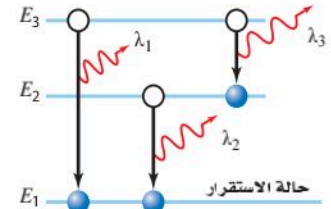
الشكل 11-4 طاقة الفوتون المنبعث تساوي الفرق في الطاقة بين مستويات الطاقة الابتدائية والنهائية للذرة.
