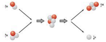
الشكل 9-6 اندماج الديوتيريوم
