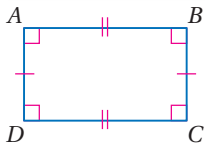
المستطيل ABCD
