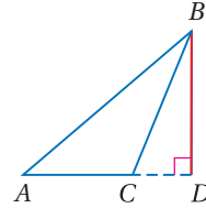
\overline{BD} هو الارتفاع من B إلى \overline{AC} .
