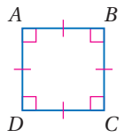
المربع ABCD
