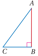
\overline{AB} هو الارتفاع إلى \overline{CB} .
